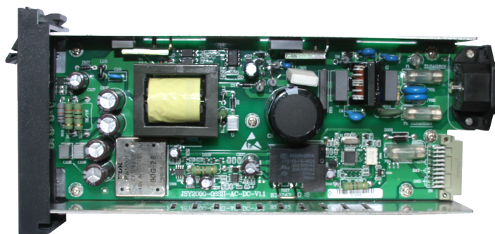
图 3-8 一次电源板
