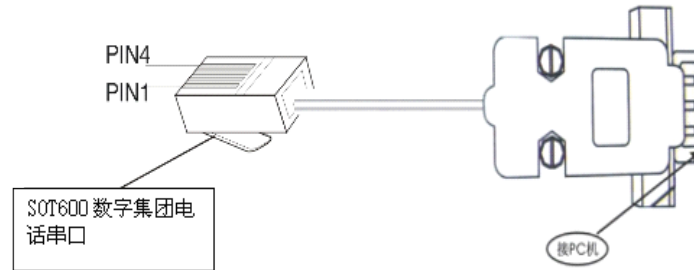
图 3-15 RS232 串口与电脑联机接口连接关系图
