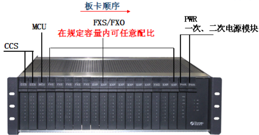
图 3-2 JSY2000-06S 机框的正面
