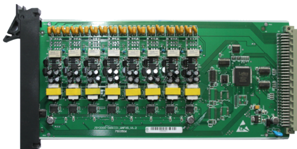
图 3-5 FXS 用户板
