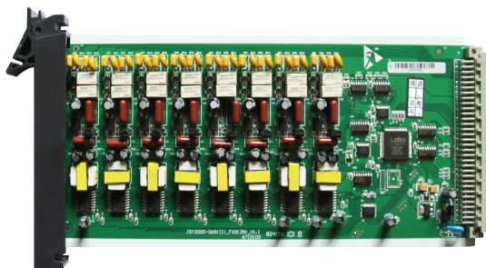
图 3-6 FXO 环路中继板
