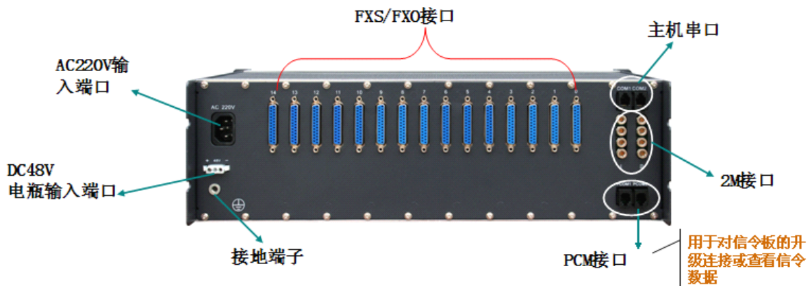
图 3-3 JSY2000-06S 机框的背面
